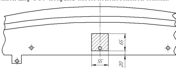
Эскиз А. Задний бампер.
